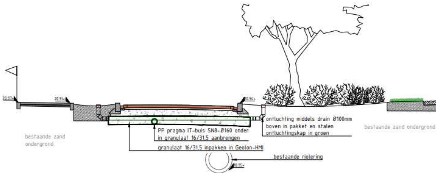
Dwarsprofiel 13-13' (Middachtenstraat 8) schaal 1:50
